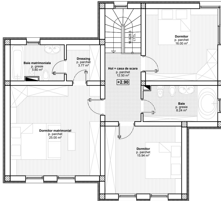
Plan etaj 112.17 mp
